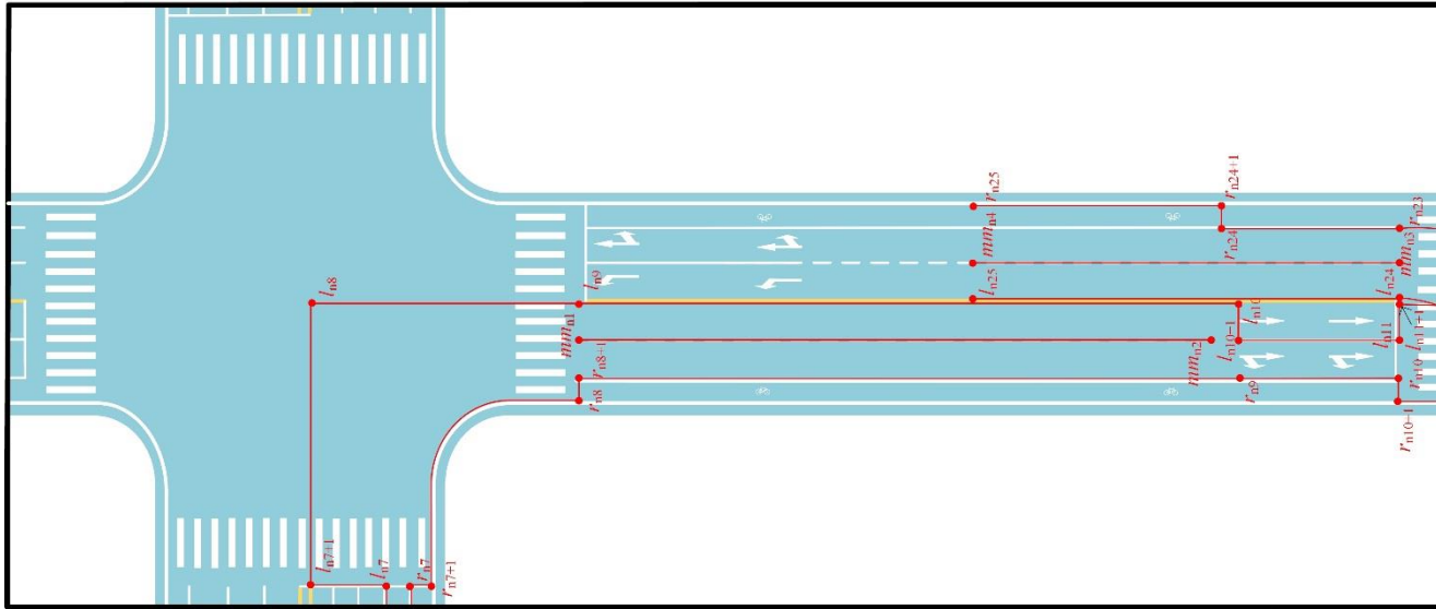
d) C区 (右转路口) 测绘点分布示意图
