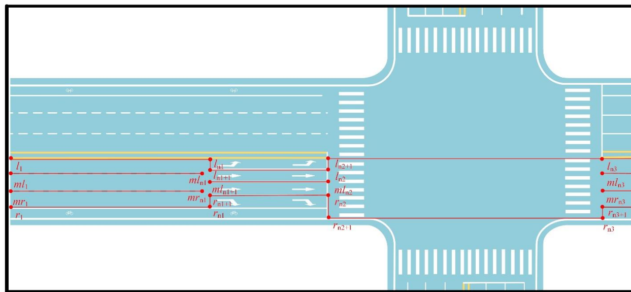
b) A区 (起点及直行路口) 测绘点分布示意图
